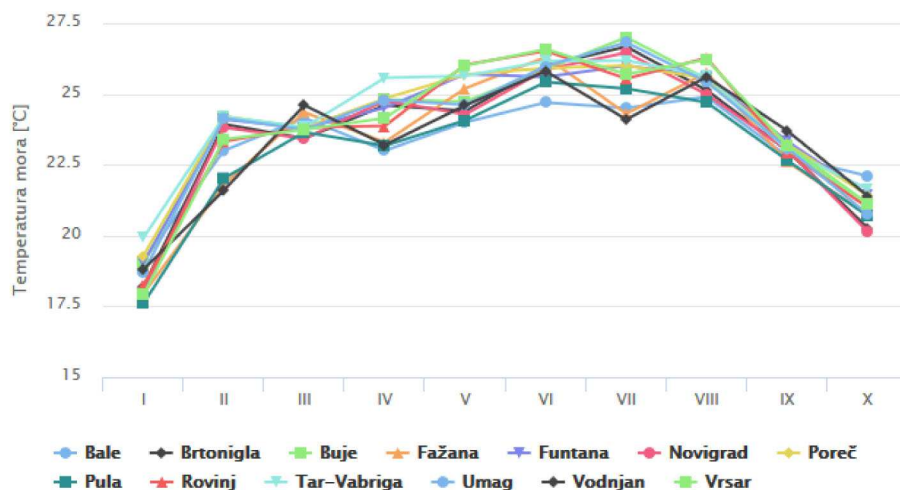
Slika br.16. Prosječne temperature mora po ispitivanjima – zapadna obala Istre
