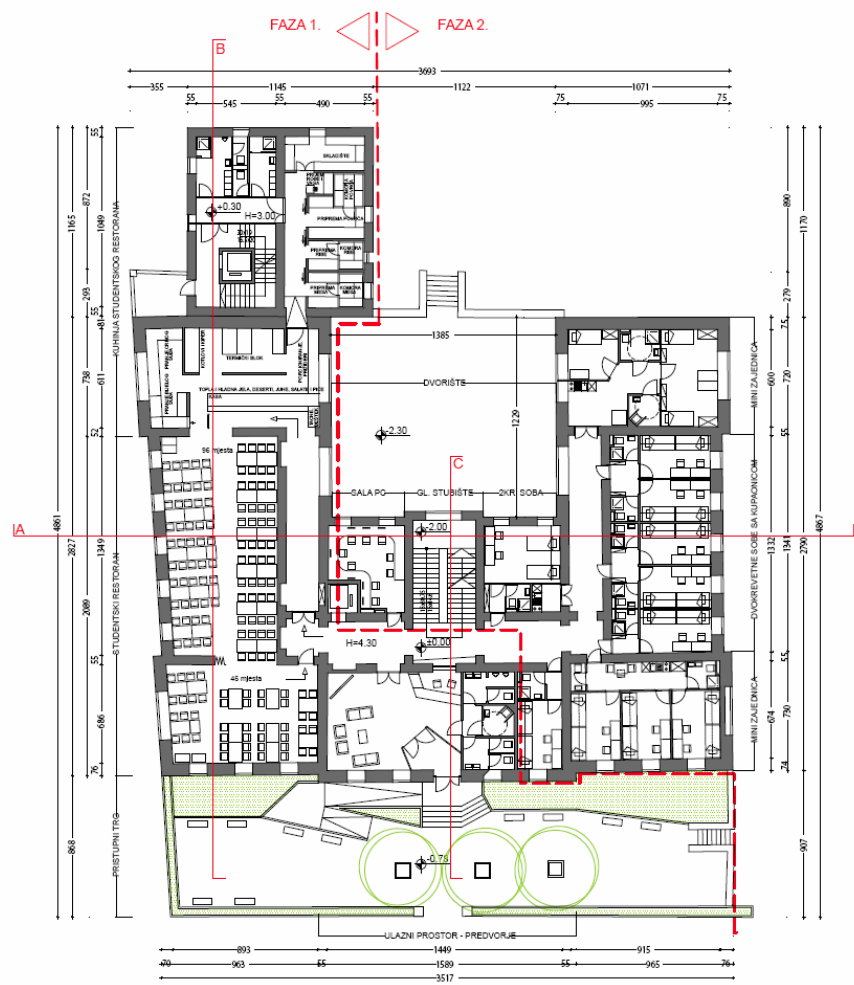
Studentski dom Pula tlocrt prizemlja
