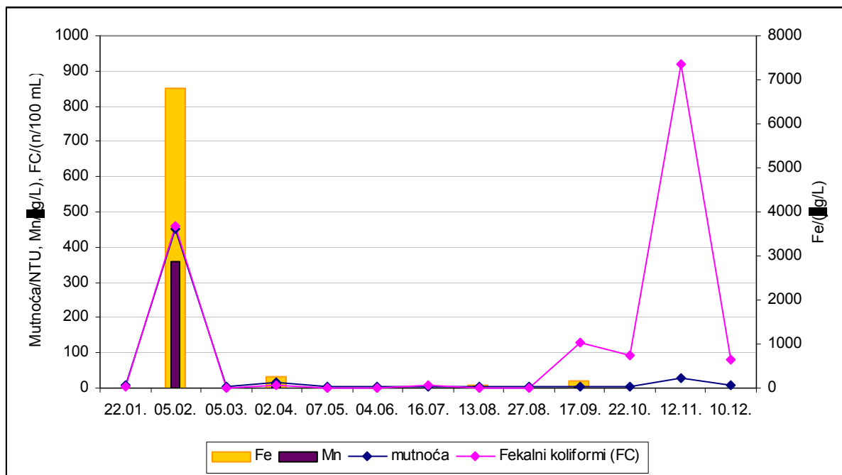
Sl.br.3. Primjer izvora Rakonek – međuovisnost pojava mutnoća i povećanih vrijednosti parametara onečišćenja (FC, Fe, Mn)
