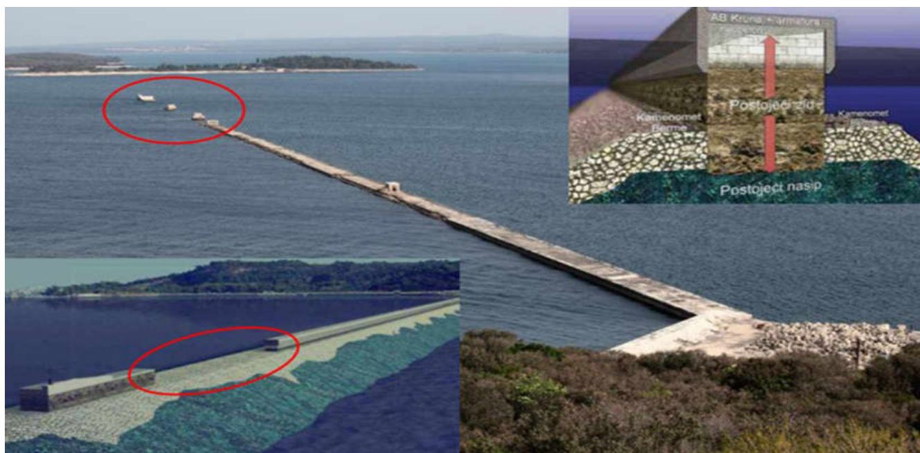
Slika 2: Prikaz lokacije i tehničkih obilježja projekta Rekonstrukcija lukobrana u luci Pula – PULA BREAKWATER
